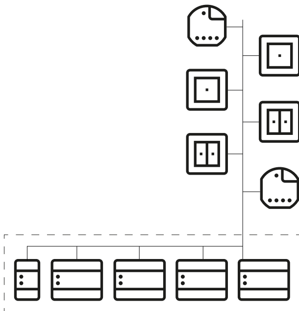
Lineare Verdrahtung
