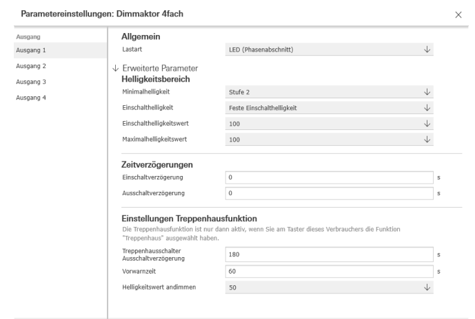
Erweiterte Parametereinstellungen des Dimmaktors
