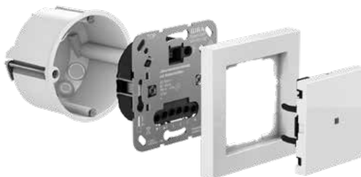
RF Multi Bedienaufsatz für KNX in Kombination mit Gira System 3000 Einsatz
