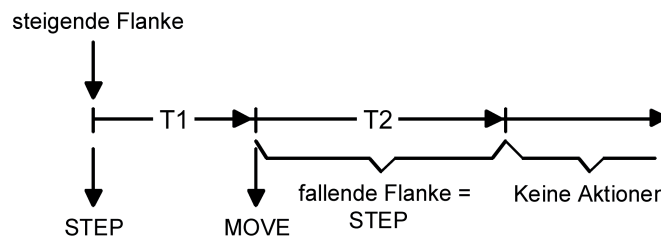
Bild 16: Bedienkonzept "Kurz-Lang-Kurz"
