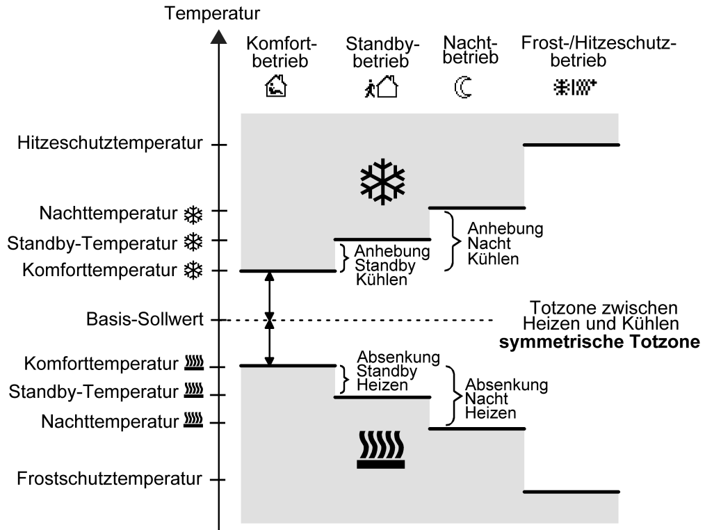
Bild 41: Solltemperaturen in der Betriebsart "Heizen und K\u00fchlen" mit symmetrischer Totzone
