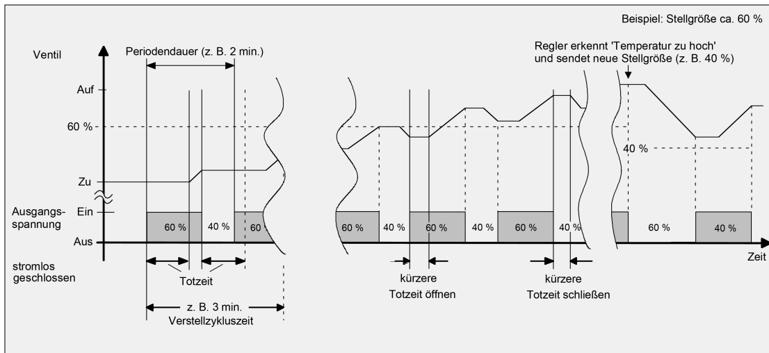
Bild 17: Idealisierter Verlauf des Ventilhubes exemplarisch dargestellt für eine Zykluszeit < Verstellzykluszeit
