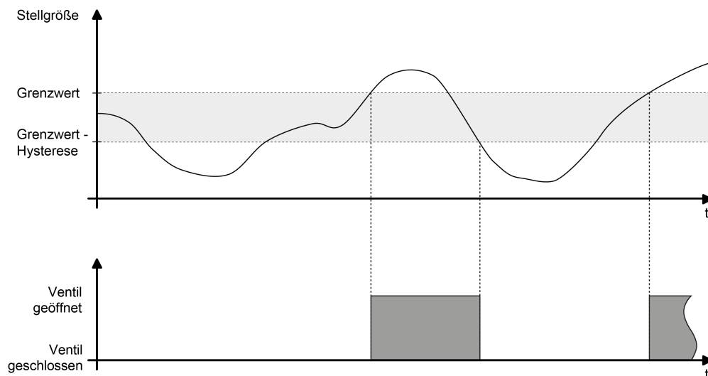
Bild 15: Beispiel einer Stellgrößenbewertung mit Grenzwert
