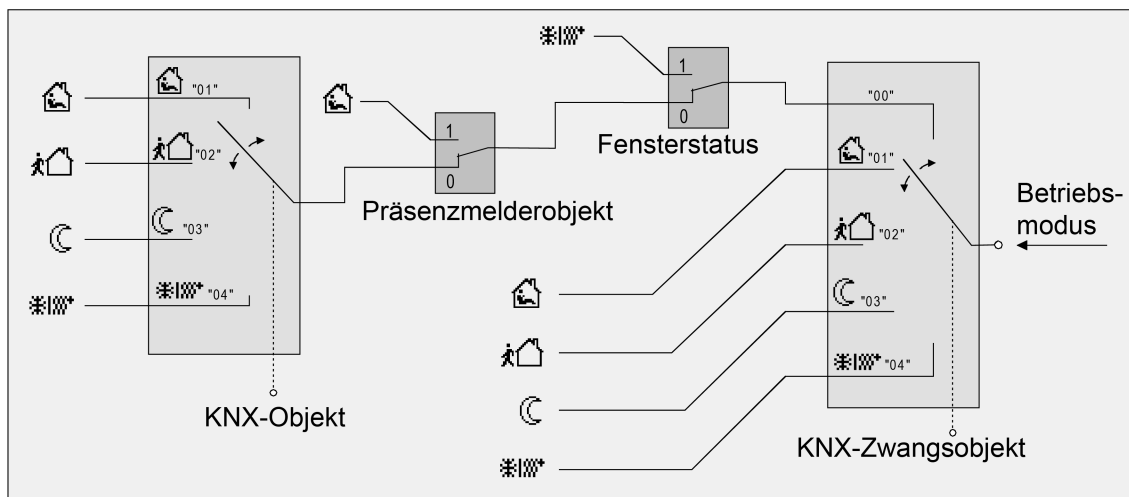
Bild 36: Betriebsmodusumschaltung durch KNX Objekt mit Präsenzmelder
