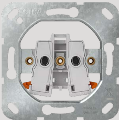
02 Steckdosen ohne Schutzkontakt und mit Steckklemme
