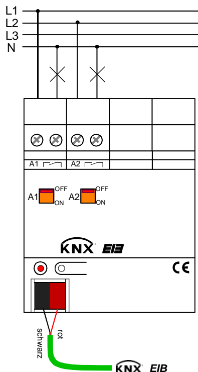
Bild 1: Elektrischer Anschluss
