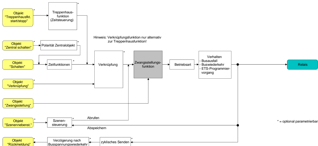
Bild 18: Funktionsschaltbild der Zwangsstellungsfunktion
