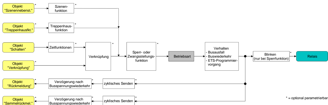
Bild 6: Funktionsschaltbild "Betriebsart"
