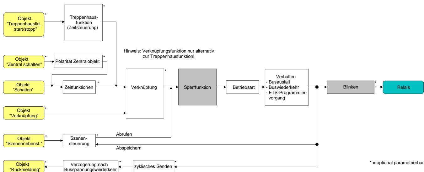
Bild 17: Funktionsschaltbild der Sperrfunktion
